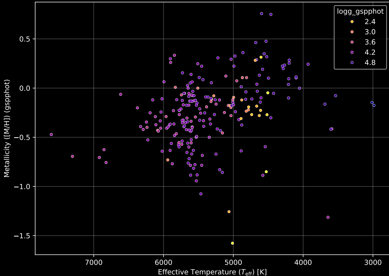
APOGEE DR17 Field: [049-52-O] Stellar Population Parameters (n= 225)
